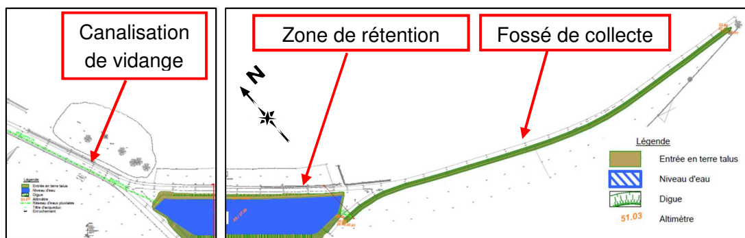
Extrait de la vue en plan projet (INGETEC – 02/06/2017)
